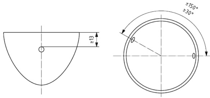
รูปที่ 16 ตัวอย่างรูเปิดที่ไม่อยู่บริเวณฐานของเล่น (ข้อ 4.4.6.1(2))
